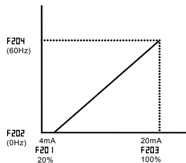
Beispiel der Einstellung der VIA Eingangsklemme (Eingangsstrom)
