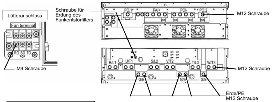
VFAS1-4500KPC
