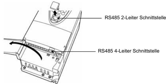
RS485 4-Leiterkommunikation
