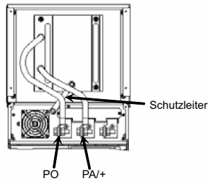
«VFAS1-2550P~2900P, 4900PC~4160KPC»
