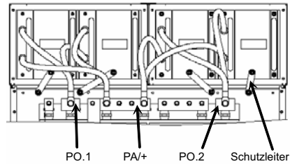
«VFAS1-4500KPC»
