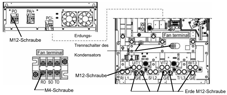
VFAS1-4355KPC, 4400KPC
