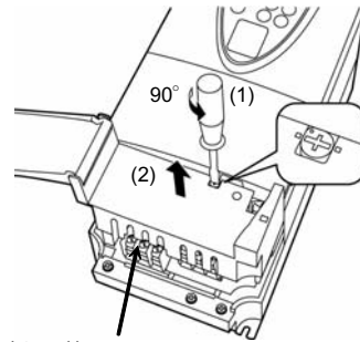
Leistungsklemmen
